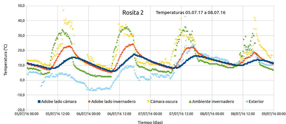
Figura 5b: registros térmicos del período 5 al 8 de julio de 2016, invernadero Rosita 2 (nuevo)
